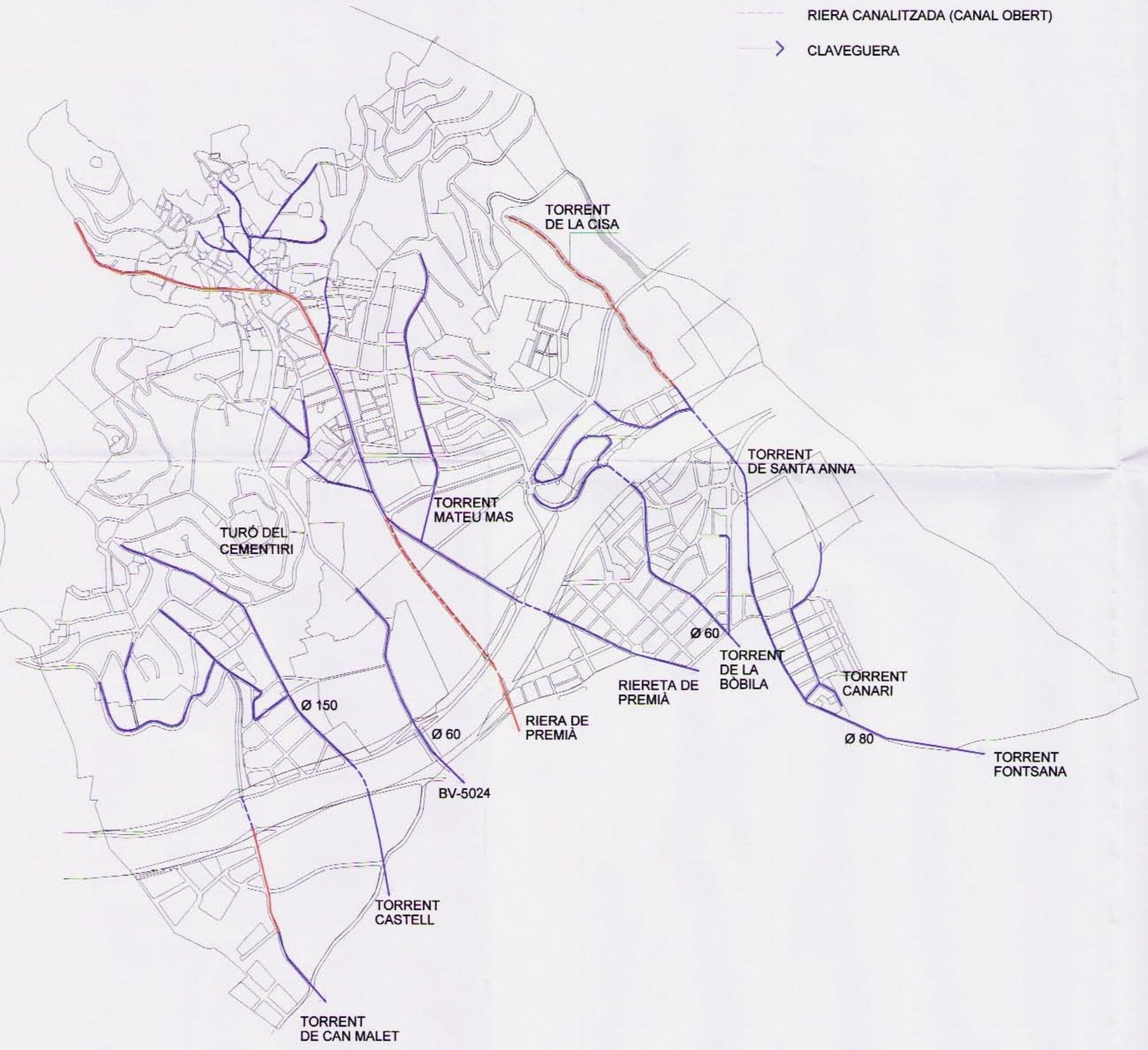
XARXA BÀSICA DEL SISTEMA DE DESGUÀS E : 1 / 10.000
