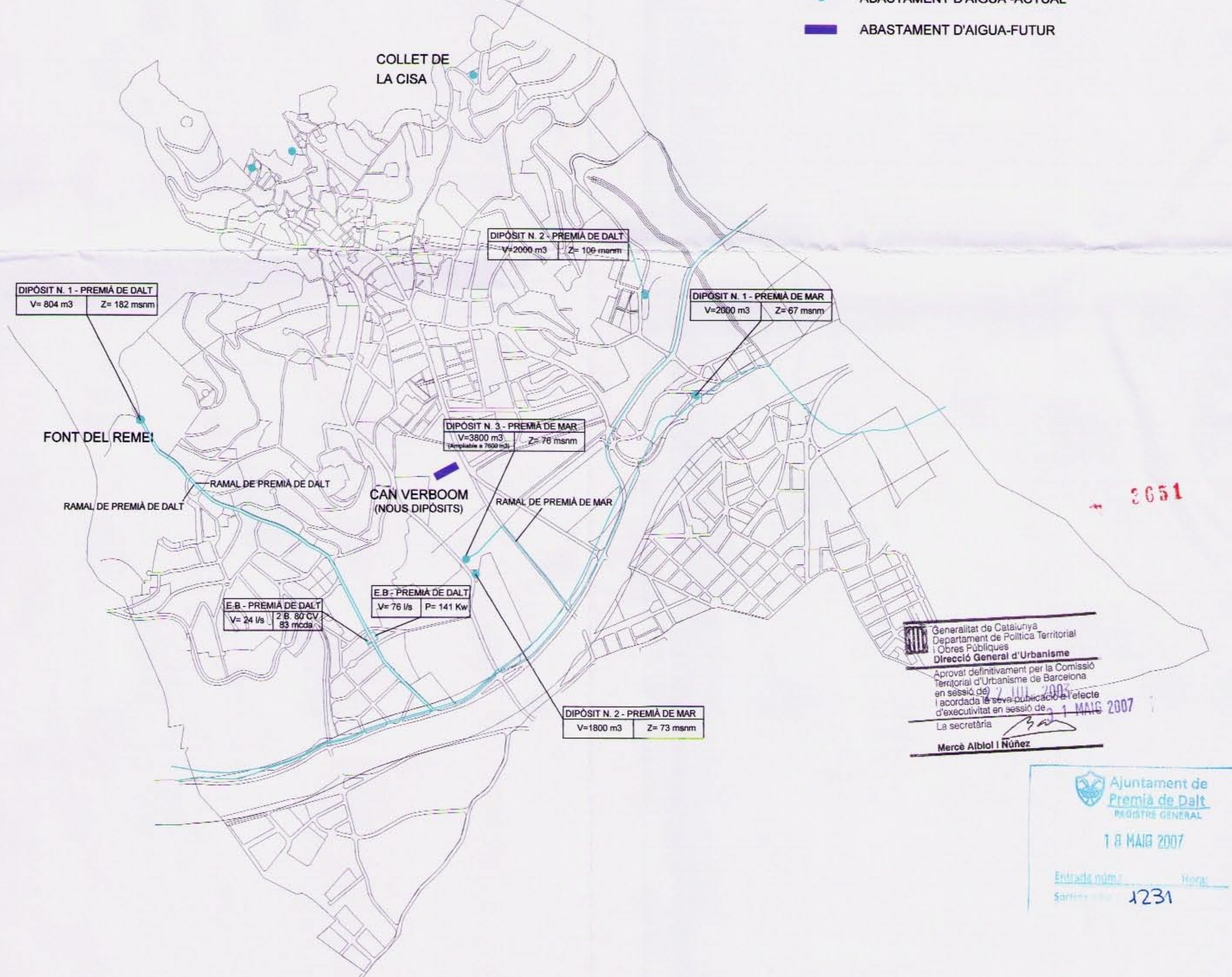
XARXA BÀSICA ABASTAMENT D'AIGUA E : 1 / 10.000
